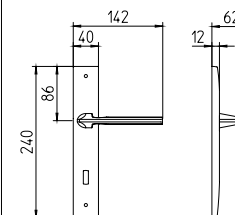
1460 con piastra on backplate
