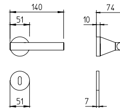
8021/M maniglia per porta senza rosetta door handle without rose
